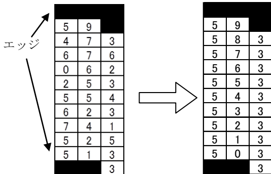
図 6 エッジ画像走査
