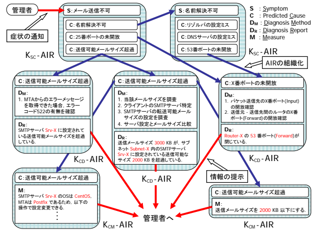
図3. K-AIRの動作例
