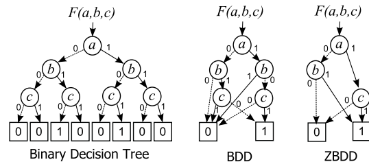
図 1: 二分決定木と BDD, ZBDD
