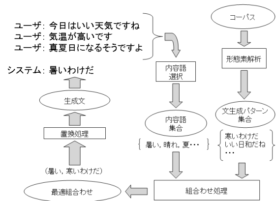
図1: 対話の流れに着目した発話生成手法
