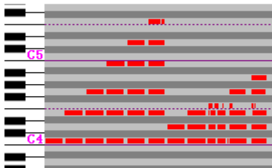
図4 実験2：音源数が未知の場合の音高推定結果
