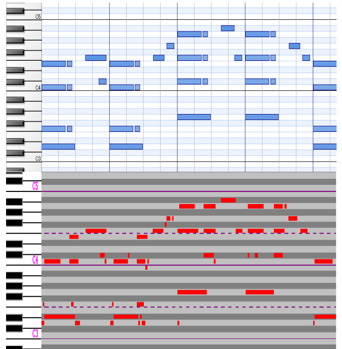
図5 実験3：楽曲サンプルデータに対する音高推定結果 (上段：正解 MIDI データ，下段：音高推定結果)
