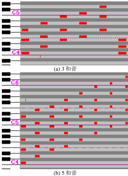
図3 実験1：音源数が既知の場合の音高推定結果
