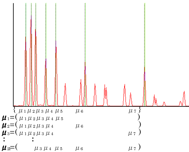
図2 複素スペクトル内挿法によるピーク検出と基本周波数候補の選択例( K = 5, L = 7 の場合)
