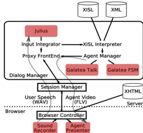
図 1 従来システムのモジュール構成
