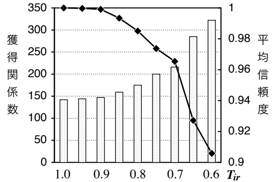
図 3: 包含率の閾値に対する獲得関係数, 信頼度の変化
