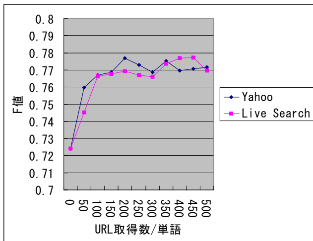
図2 URL取得数による推定性能の変化
