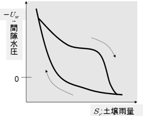
図 2: 一般的な降雨特性曲線
