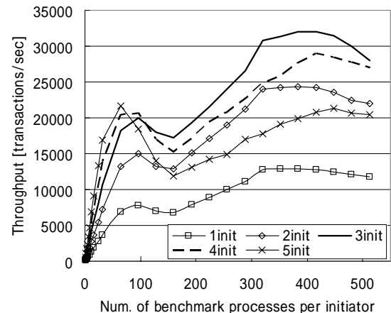
図 1: 高負荷 IP-SAN システムの性能
