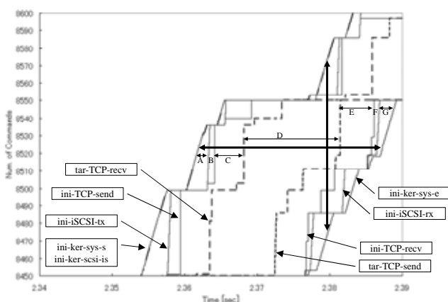
図 4: 4 イニシエータ 140 プロセス時動作解析
