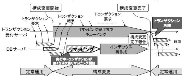
図 4: トランザクション管理方式
