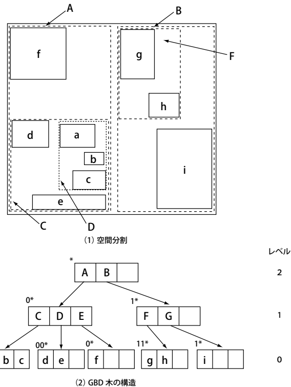
図 1: GBD 木の概要
