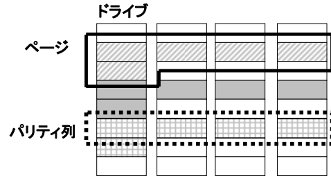
図4 容量プールをページで分割する例
