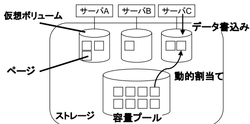
図1 動的容量割当て機能
