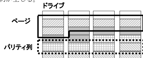
図2 同一パリティ列内に複数ページが混在する例
