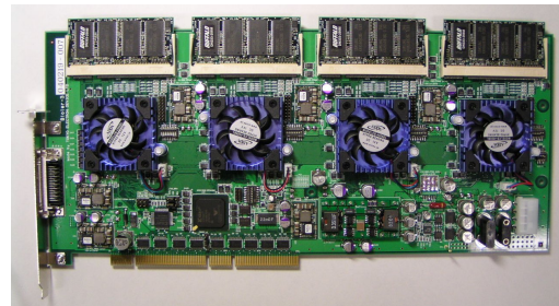
図 2: Bioler-3 概観図。
