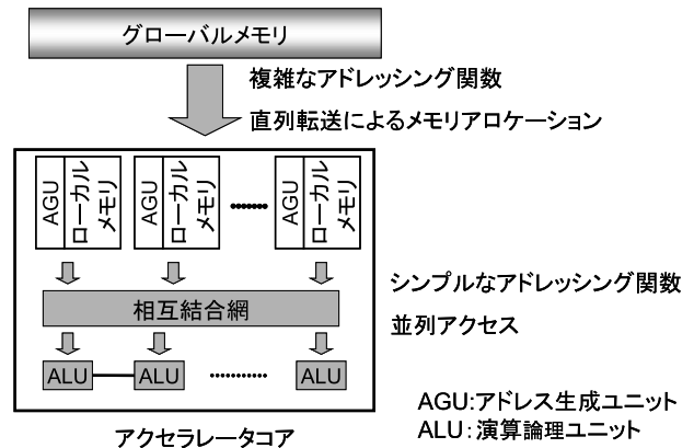
図1: ヘテロジニアスマルチコアの構成
