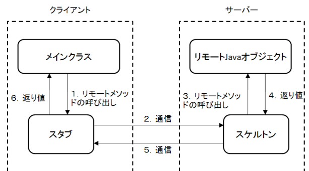
図 1 Java RMI の動作
