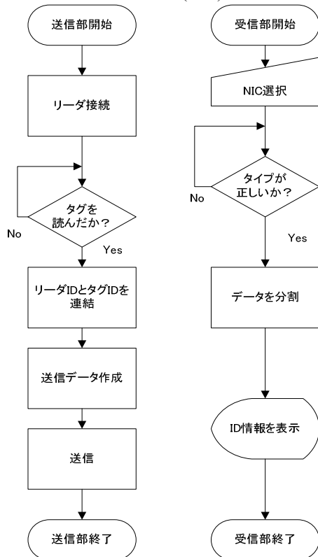
図4 動作概要
