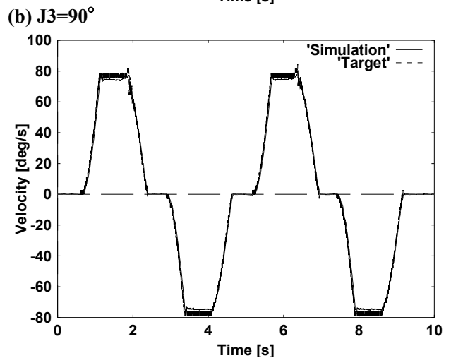
図4 シミュレーション結果及び制御対象測定結果 (a) 角変位：モデルと制御対象の比較 (b) 角速度：モデルと制御対象の比較
