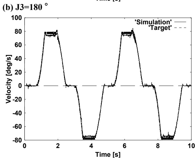
図3 シミュレーション結果及び制御対象測定結果 (a) 角変位：モデルと制御対象の比較 (b) 角速度：モデルと制御対象の比較
