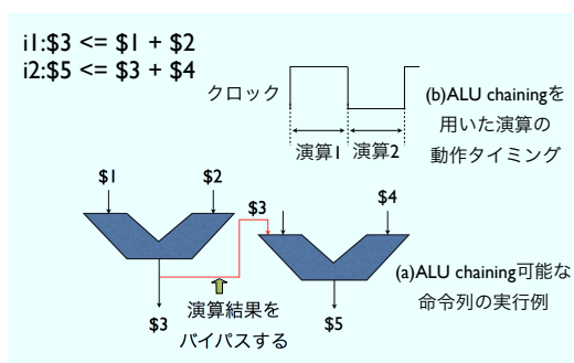
図 1: ALU chaining の仕組み
