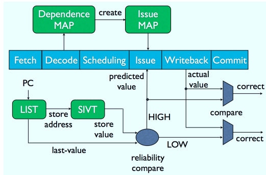
図2: 提案手法を適用したパイプライン
