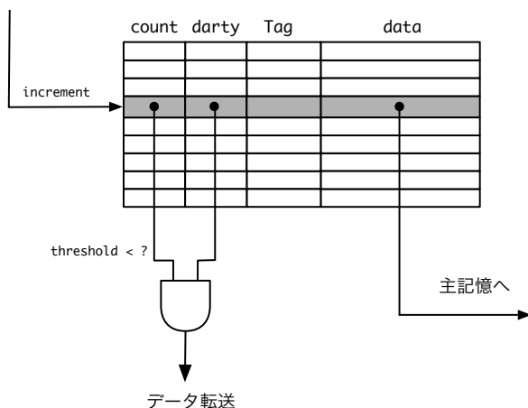
図3 提案機構
