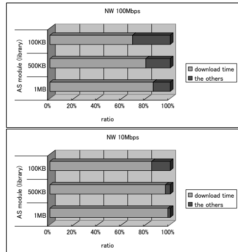
図 4: 動的ダウンロード時間の比率
