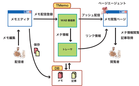
図 1: TMemo の構成
