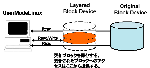
図 1 Layered Block Device による COW の実装
