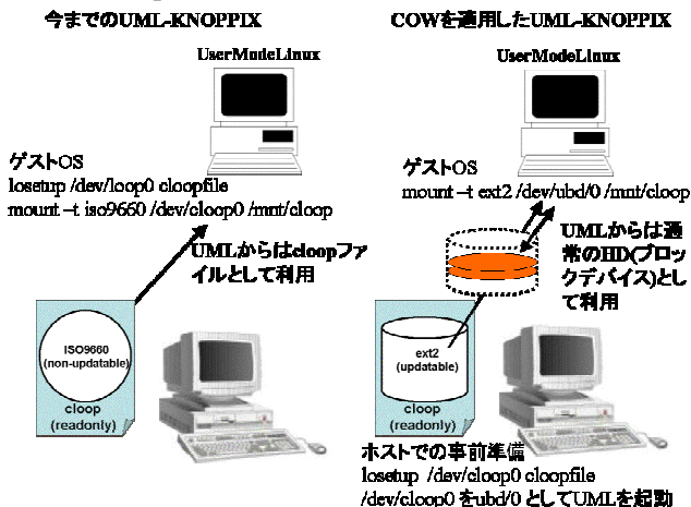
図 3 COW 適用前後の UML-KNOPPIX の実装
