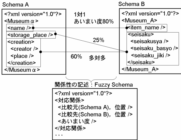
図2 Fuzzy Schema
