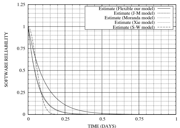
図3：一般化ハザードレートモデルに対する推定されたソフトウェア信頼度。
