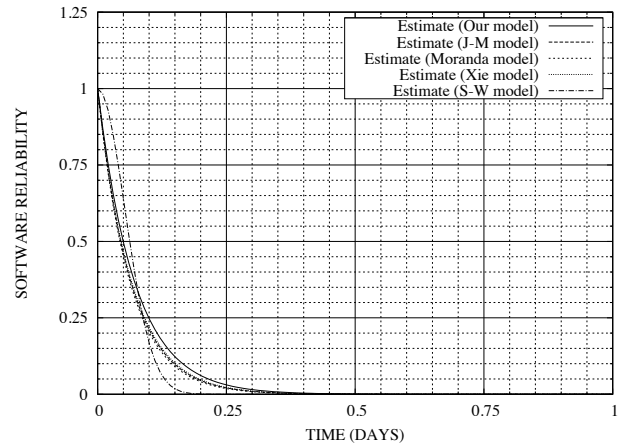
図1：ハザードレートモデルに対する推定されたソフトウェア信頼度。
