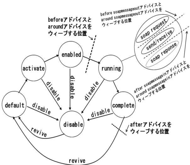
図2 アドバイスの織り込み位置
