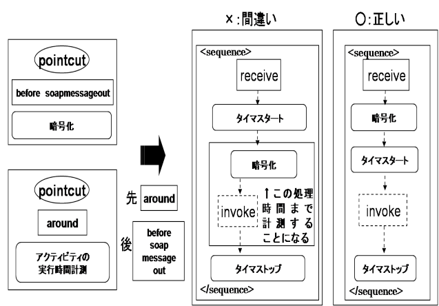
図7 順番を再定義する必要性
