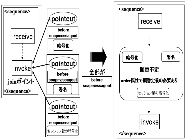
図6 「アドバイスタイプが同一であるアドバイス間の干渉」の発生
