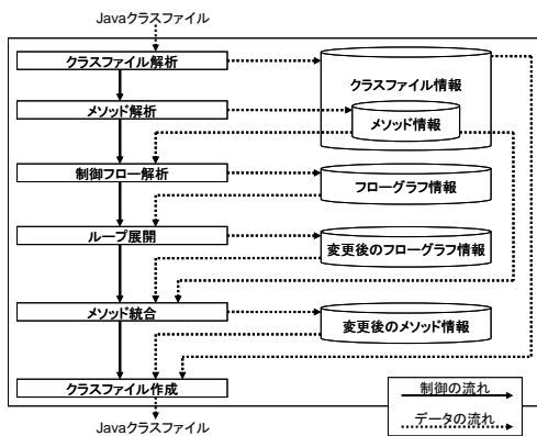
図-1 本システムの全体構造
