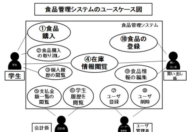
図 1：基本機能を実装したシステムのユースケース図
