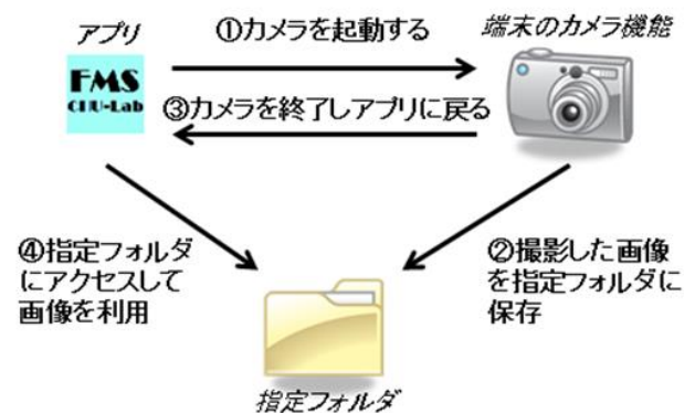
図 5: 外部カメラアプリ利用の仕組み
