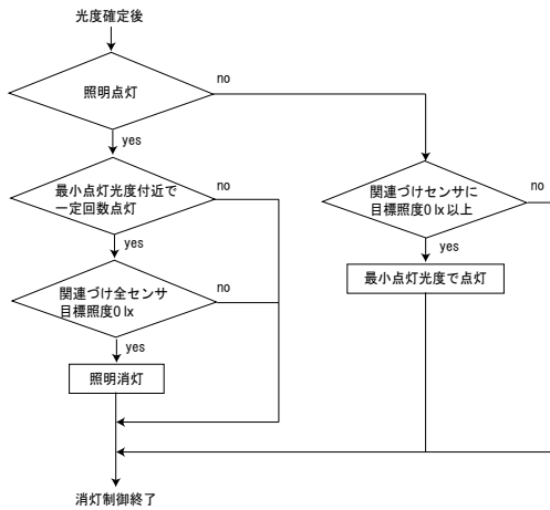
図1: 消灯アルゴリズム
