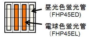
図2: 試作機の概略図
