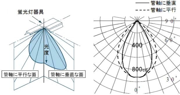
図 3: 空間的な配光データ 図 4: 試作機の配光データ (ランプ光束 1000[lm])
