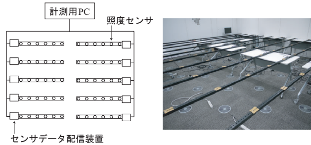
(a) 照度分布計測システムの構成
