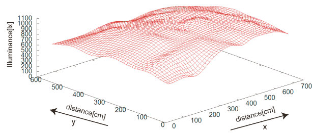
図 3: 均一光度環境における実験結果
