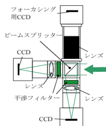
図4 装置図
