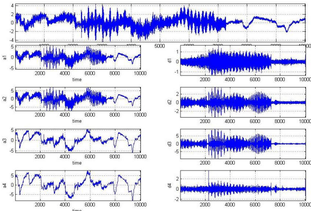
図2 原信号と各ウェーブレット変換係数
