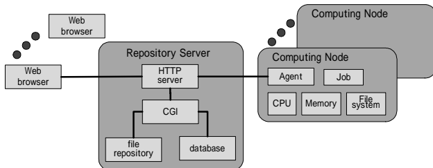
図 1 ShareTask の構成
