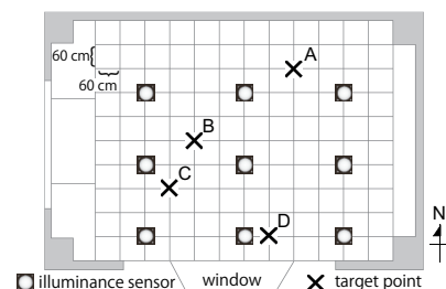
図1: 実験環境
