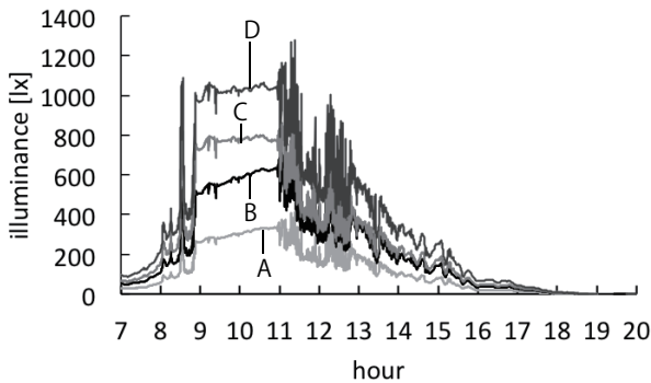
図2: 実測照度値
