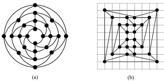
図1: (a) 4連結 p-5-k 重ドーナツグラフ G(p=4, k=4) , (b) G の格子直線描画。
