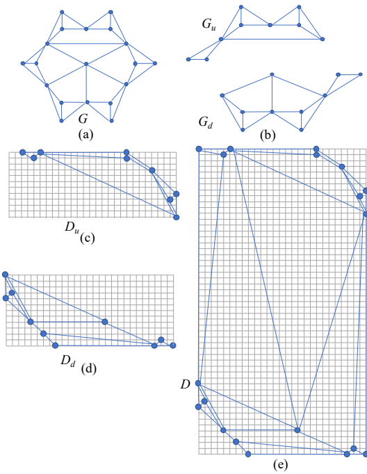
図 1: (a) 平面グラフ G , (b) グラフ G_u および G_d , (c) G_u の描画 D_u , (d) G_d の描画 D_d , (e) G の描画 D .
