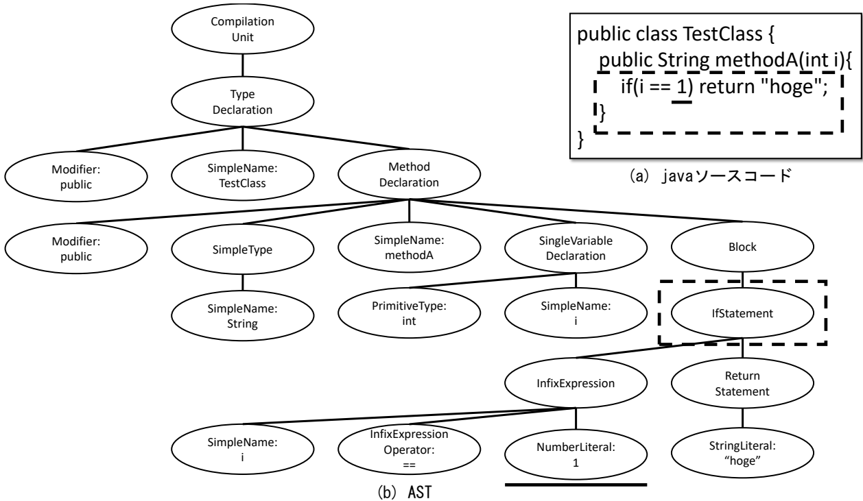
図 1: ソースコードと AST
