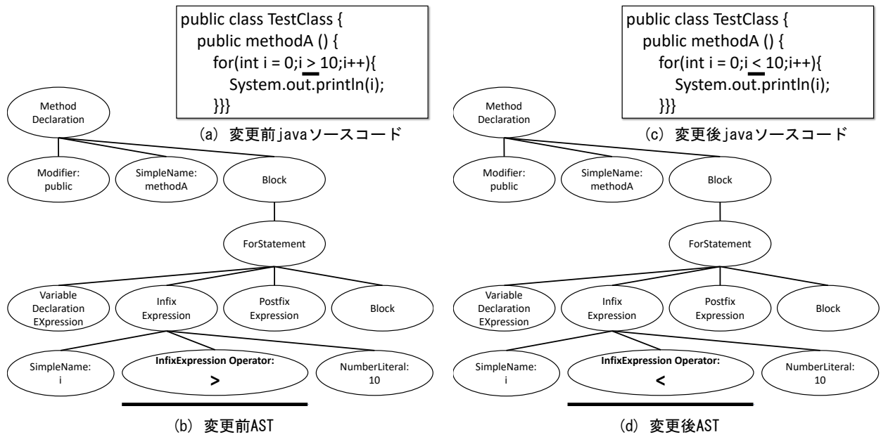
図 4: 変更前後のソースコードと AST
