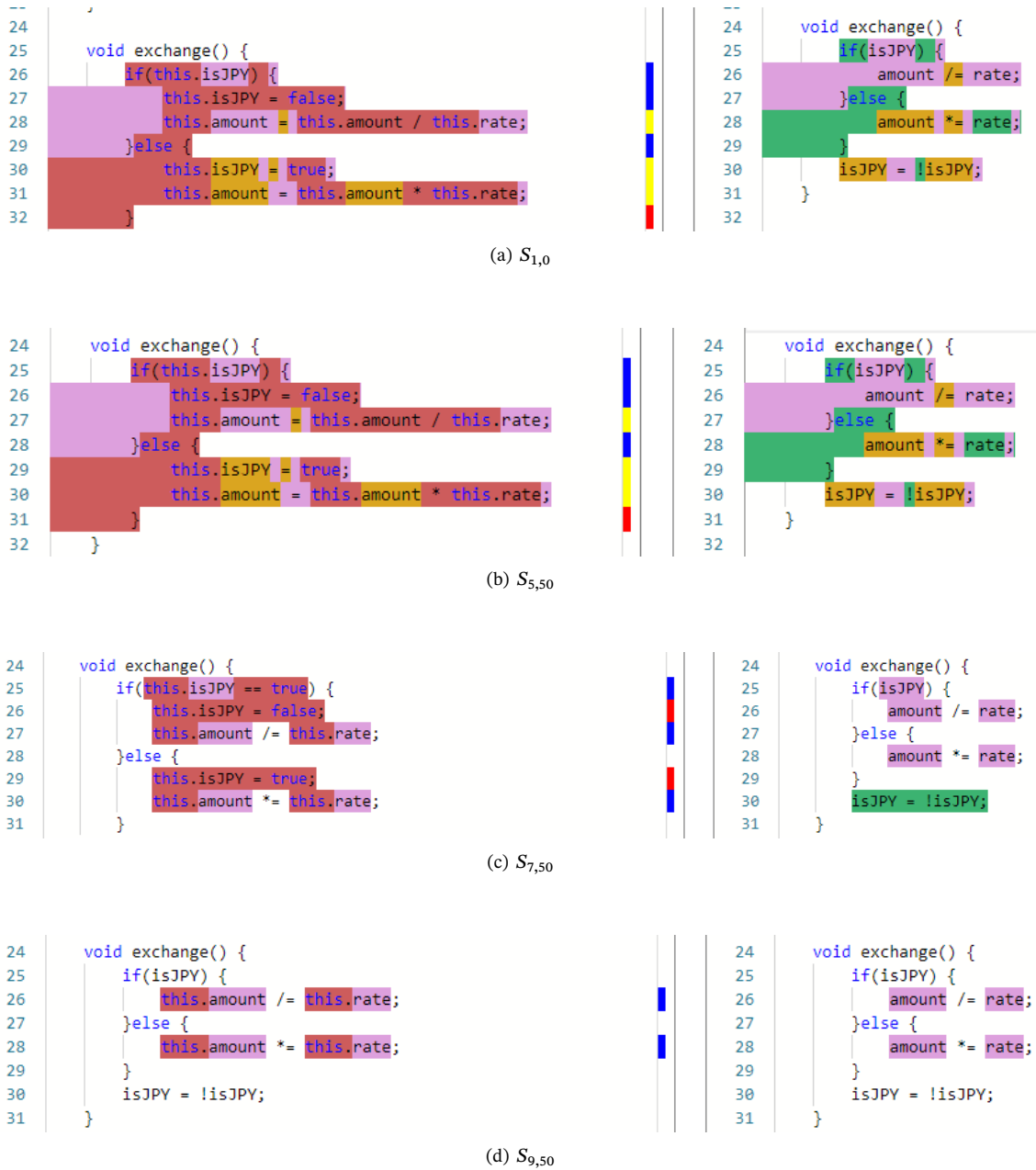
図 6: exchange メソッドの変更履歴
