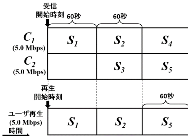
図2 単純手法の配信スケジュール例
