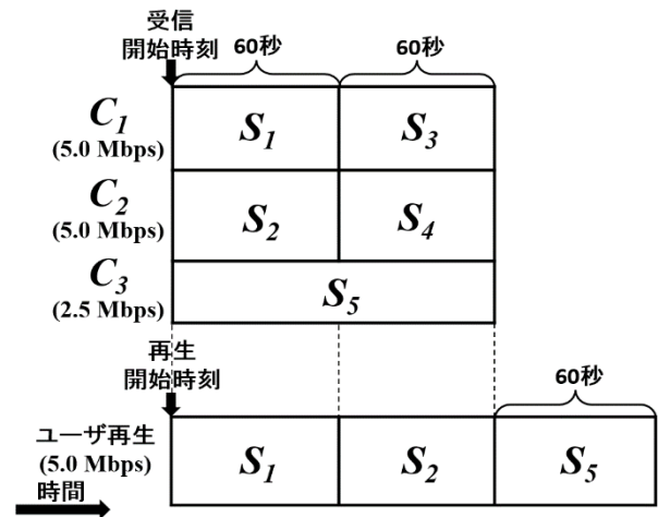
図3 CCB法の配信スケジュール例
