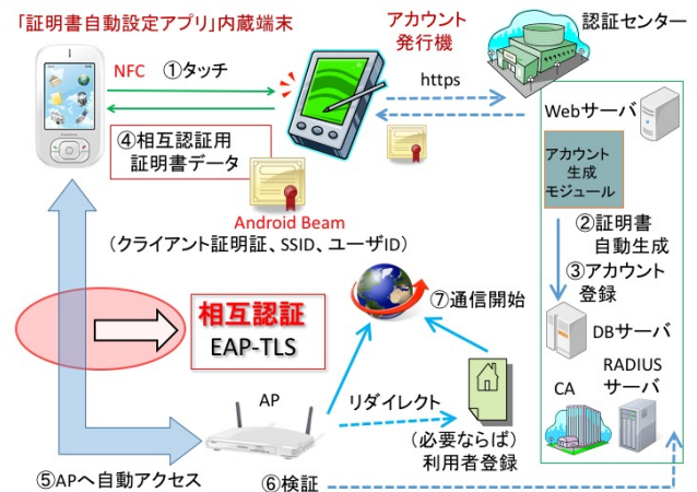
図3：ユーザーアカウントプロビジョニングシステムの構成
