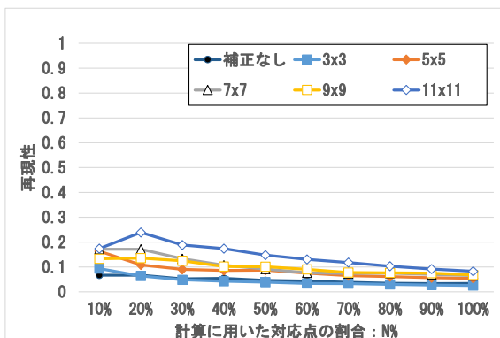
図 21 事前にメディアンフィルタを用いた img1 と img6 における SIFT の再現率
