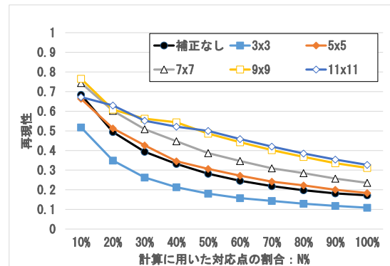
図 23 事前にコントラストとノイズを補正した場合の img1 と img2 における再現率
