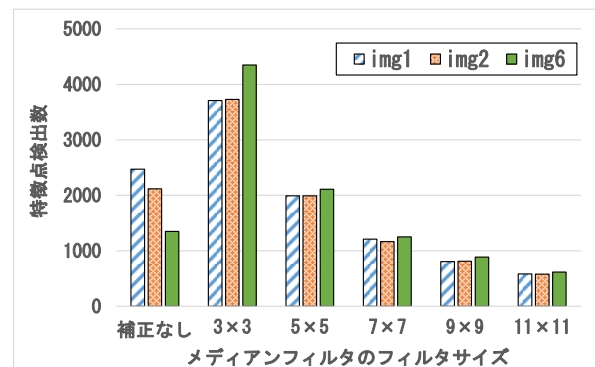
図 22 事前にコントラストとノイズを補正した場合の SIFT の特徴点検出数
