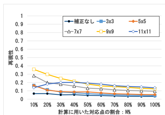
図 24 事前にコントラストとノイズを補正した場合の img1 と img6 における再現率
