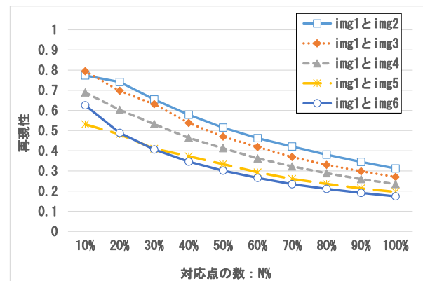
図16 上位N%を用いた提案手法の再現性
