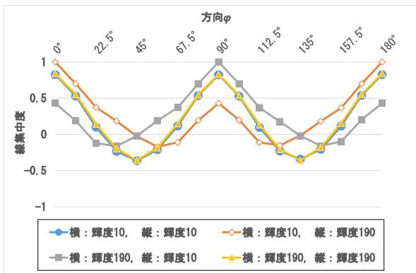
図 5 線の交差箇所における方向ごとの線集中度
