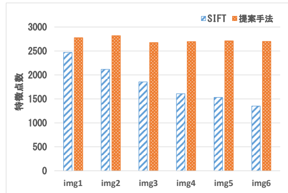
図13 各画像で検出した特徴点数
