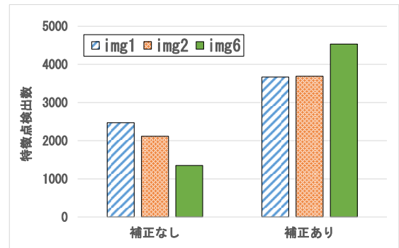
図17 事前にコントラストを補正した場合のSIFTの特徴点検出数
