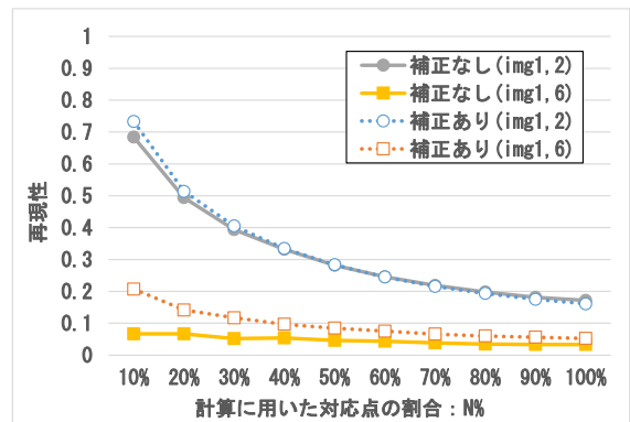
図18 事前にコントラストを補正した場合のSIFTの再現性
