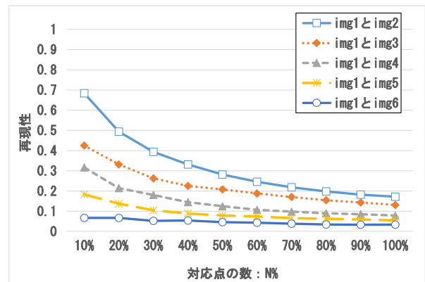
図15 上位N%を用いたSIFTの再現性
