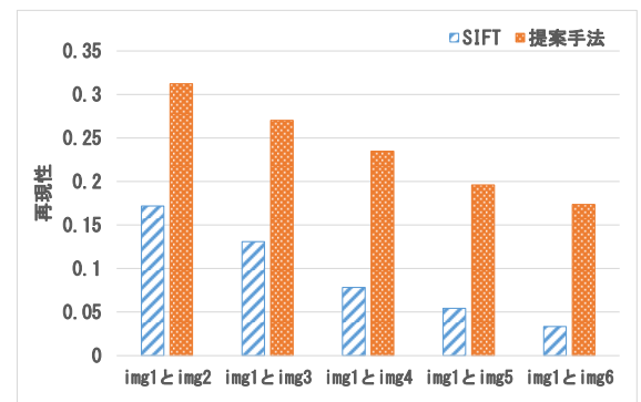
図14 再現性の比較
