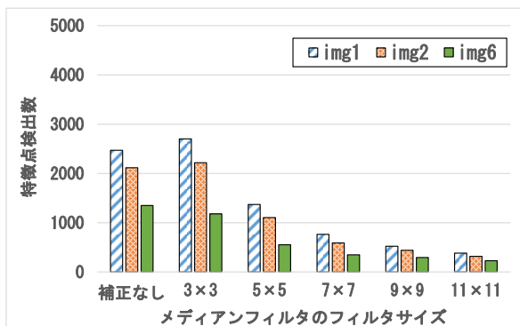
図 19 事前にメディアンフィルタを用いた場合の SIFT の特徴点検出数
