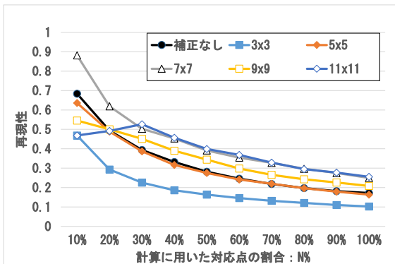
図 20 事前にメディアンフィルタを用いた img1 と img2 における SIFT の再現率
