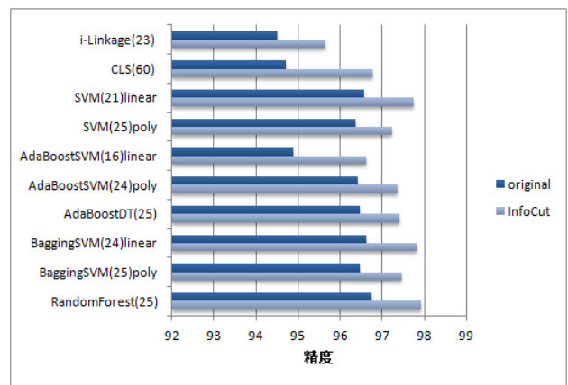
(b)精度
