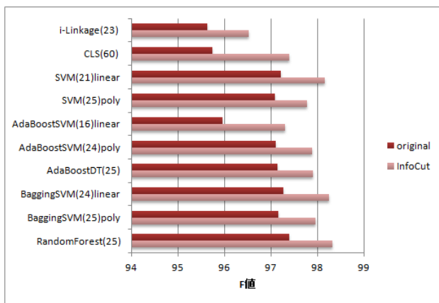
(a)F 値
