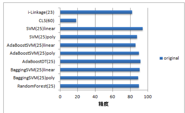
(b)精度
