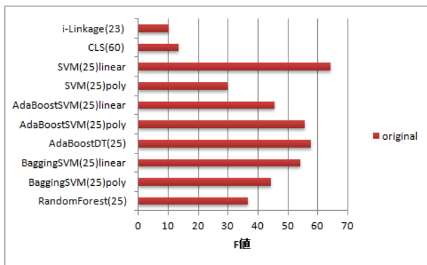
(a)F 値
