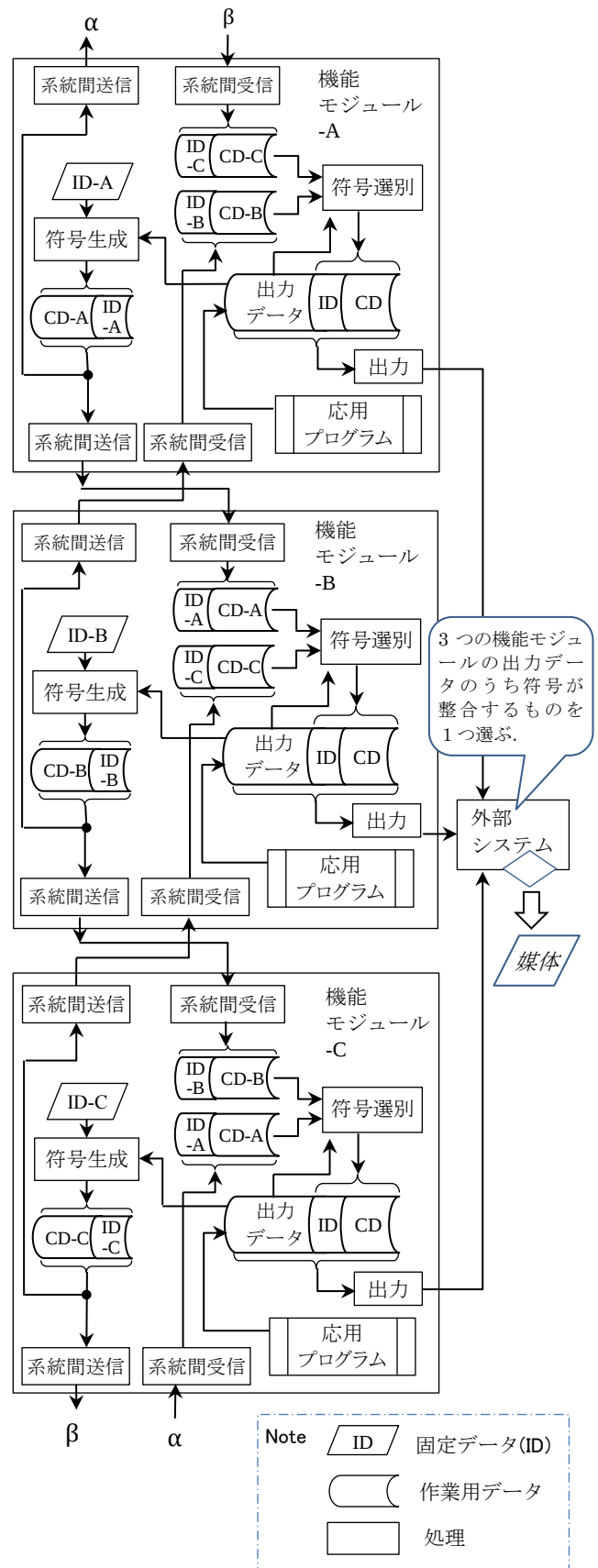
図6 データと符号を媒体に記録する高信頼性システムの構成例
