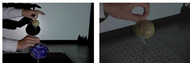
図6：満月の様子
