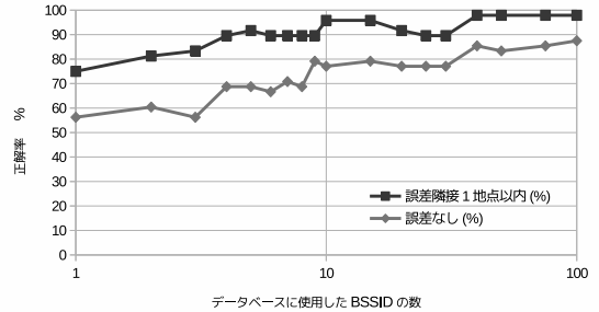
図 3: データベースで使用する BSSID ごとの正解率のグラフ
