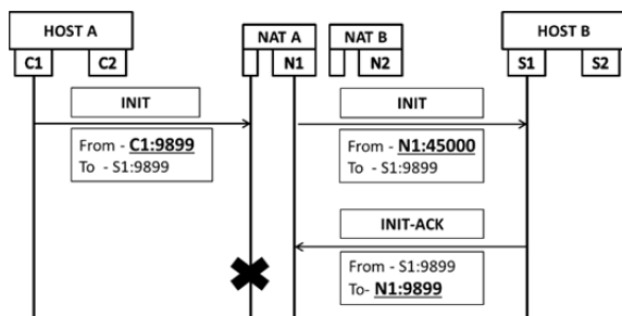
図3 FreeBSD カーネルの SCTP 実装での UDP ポート番号
