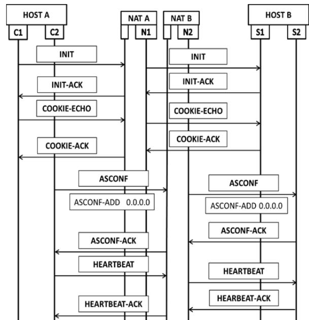
図 2 正常な SCTP 処理フロー
