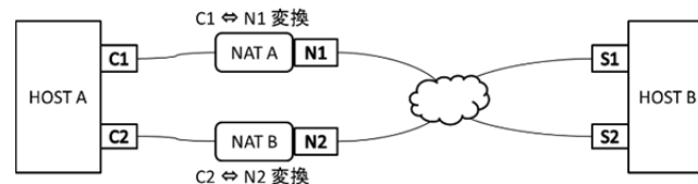
図 1 想定するネットワーク構成
