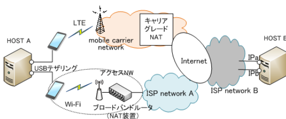
図4 実験ネットワーク
