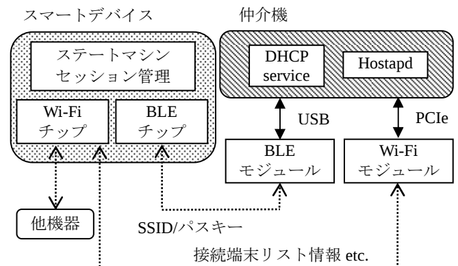
図2 プロトタイプの HW/SW 構成
