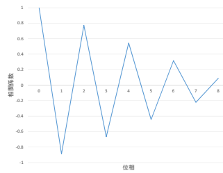
図2 自己相関サンプル
