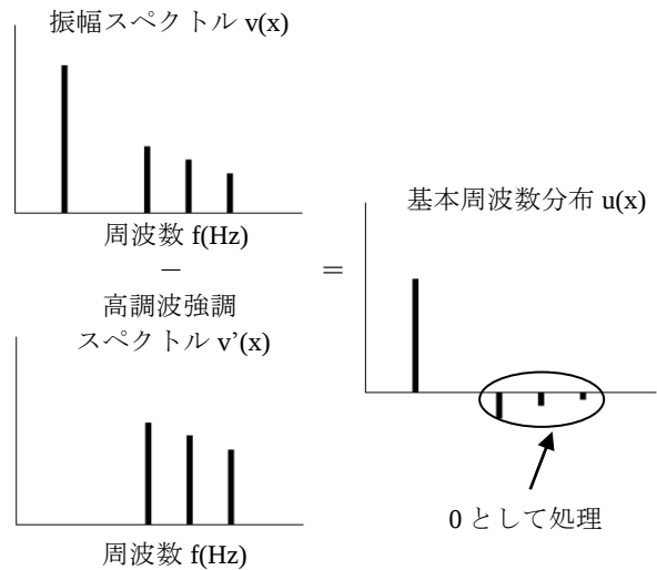
図3 高調波強調スペクトルの減算
