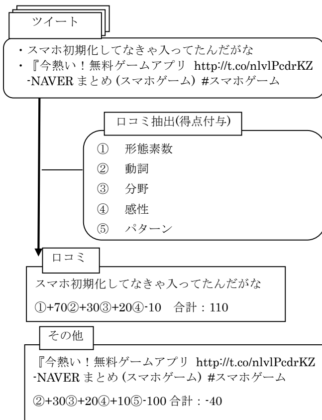
図 1 ロコミ情報抽出の流れ
